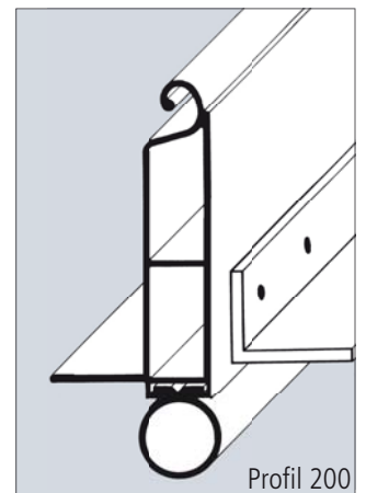
Schlusschiene Profil 200 mit angenietetem Aluwinkel
