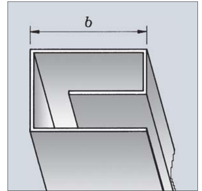
Sturankerführungen aus Stahl Tiefe der Rolltorbreite entsprechend von 80-250 mm
